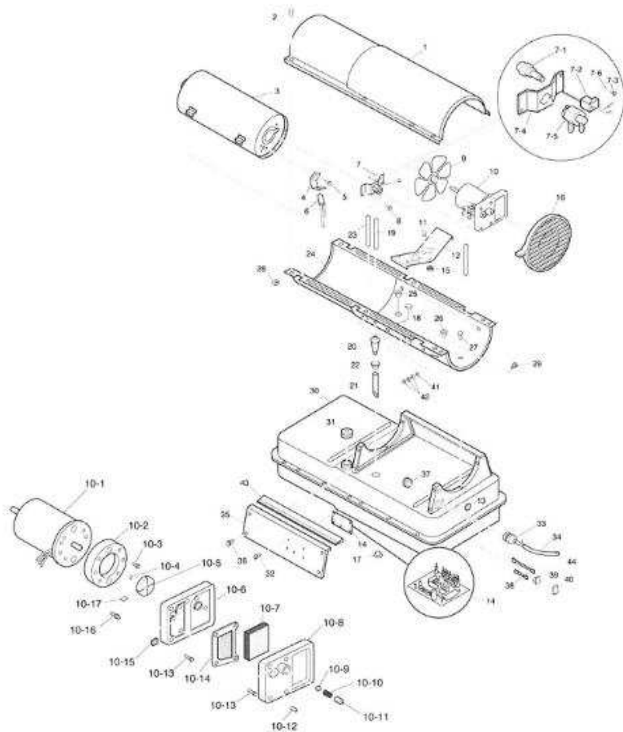
Conjunto Motor-Bomba
